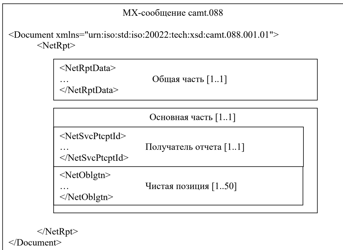
Рисунок 1 – Структура МХ-сообщения camt.088
